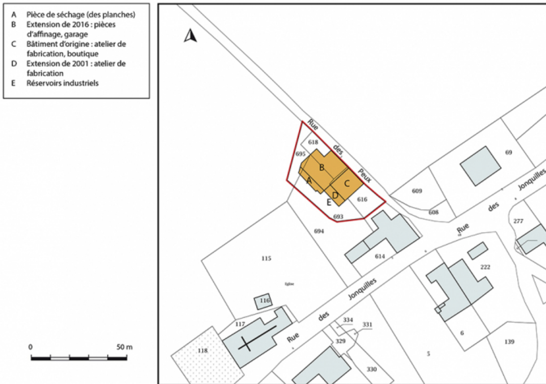
Plan-masse et de situation. Extrait du plan cadastral, 2018, section A. 25, Grand'Combe-des-Bois, 3 rue des Peux
