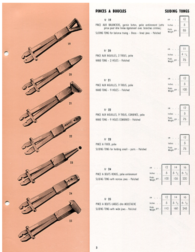
Catalogue L.H.T. 4. [catalogue de production p. 3 : pincettes à boucles], [3e quart 20e siècle]. 25, Montécheroux
