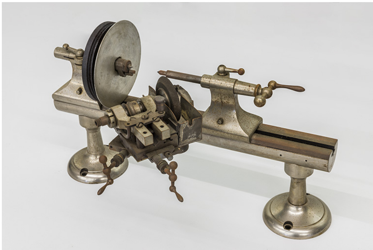
Touret d'affûtage (1957).
