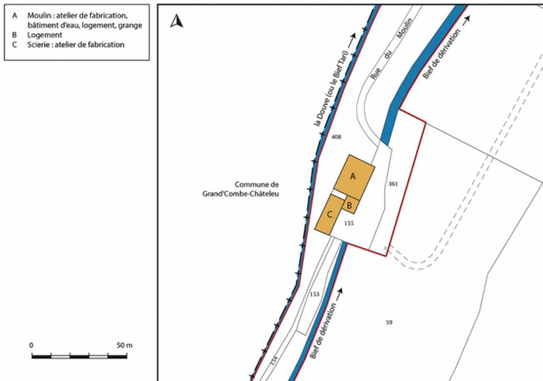
Plan-masse et de situation. Extrait du plan cadastral, 2016, section A, 1/2 500 agrandi à 1/1 000. 25, Montlebon, 17 rue du Moulin, lieudit : Cornabey
