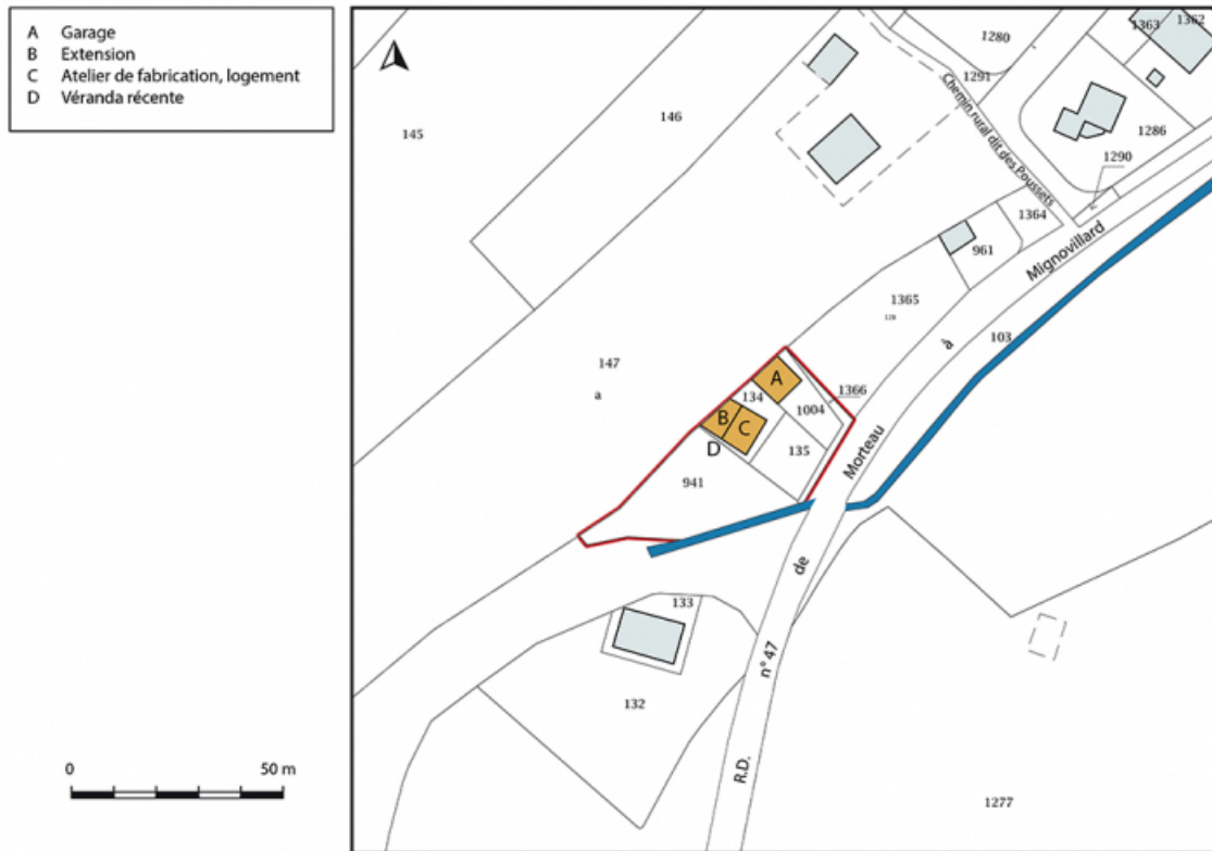
Plan-masse et de situation. Extrait du plan cadastral, 2017, section B, 1/2 500 agrandi à 1/1 000. 25, Grand'Combe-Châteleu, lieudit : le Bas de la Fin
