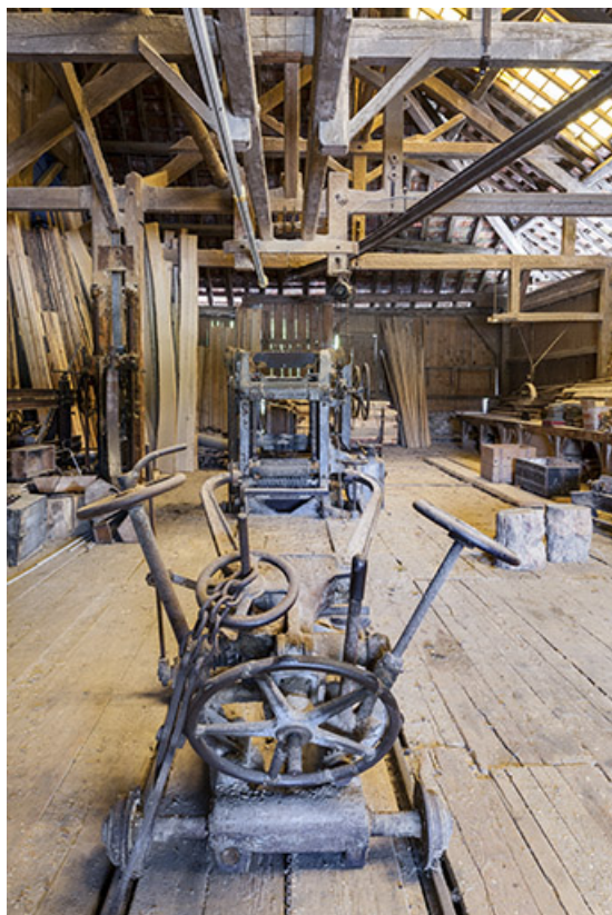
Châssis multilames et son chariot. Vue axiale. 25, Labergement-Sainte-Marie, 5 rue de Mouthe
