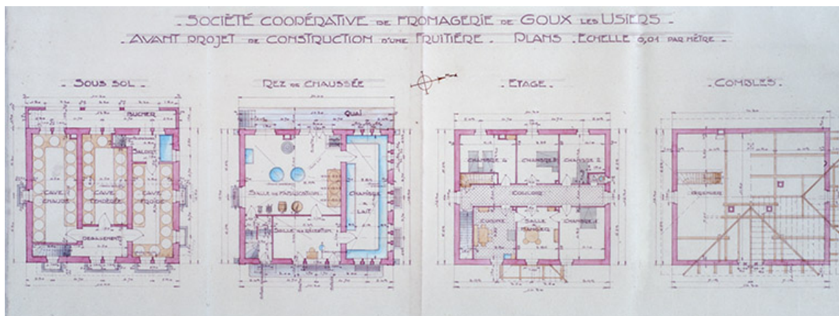
Société coopérative de fromagerie. Avant-projet de construction d'une fromèrie - Plans, 1929. 25, Goux-les-Usiers, 23 rue des Ecoles
