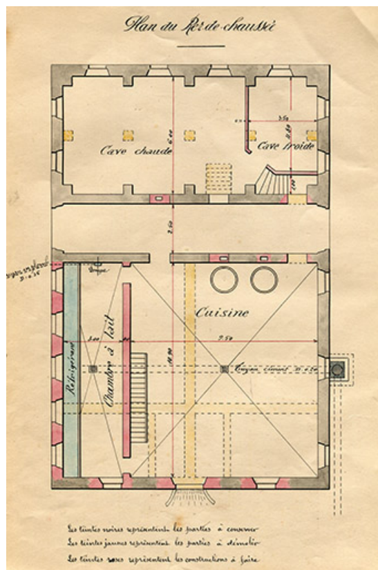
Transformation et réfection du chalet. Plan du rez-de-chaussée, 1902.
