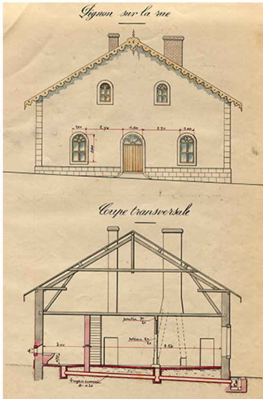
Transformation et réfection du chalet. Pignon sur rue et coupe transversale, 1902. 25, Courvières, 1 rue de Cuvier
