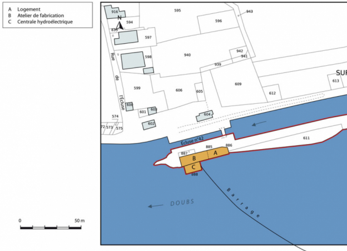
Plan-masse et de situation. Extrait du plan cadastral, 2015, section A. 25, Ougney-Douvot, lieudit : Ougney-les-Champs
