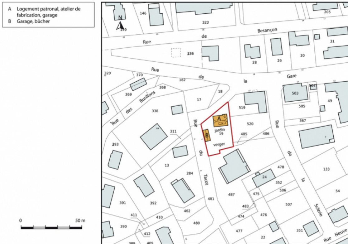
Plan-masse et de situation. Extrait du plan cadastral, 2015, section AI. 25, Charquemont, 1 rue du Tacot
