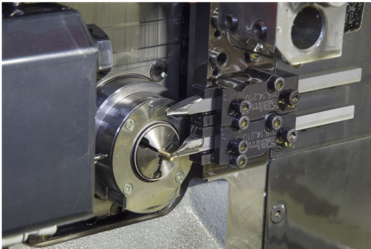
Machine à décolleter récente : pièce et outils. 25, Charquemont, 18 rue de Besançon
