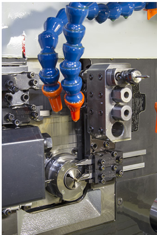
Machine à décolleter récente : installation de lubrification de la pièce et des outils. 25, Charquemont, 18 rue de Besançon
