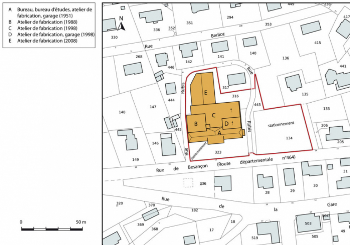
Plan-masse et de situation. Extrait du plan cadastral, 2015, section AB. 25, Charquemont, 18 rue de Besançon
