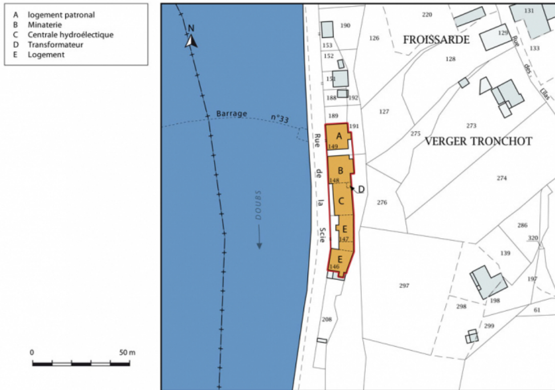
Plan-masse et de situation. Extrait du plan cadastral, 2015, section D. 25, Chaux-lès-Cerval, 14, 16 rue de la Scie, lieudit : Verger Tronchot
