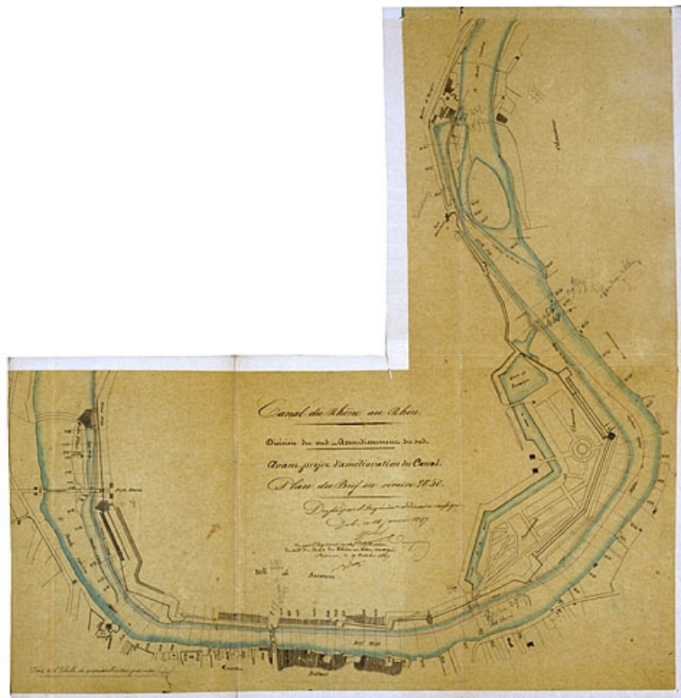
Avant-projet d'amélioration du canal. Plan du bief en rivière n° 50 [du moulin Saint-Paul au moulin de Tarragnoz], 1847. 25, Besançon
