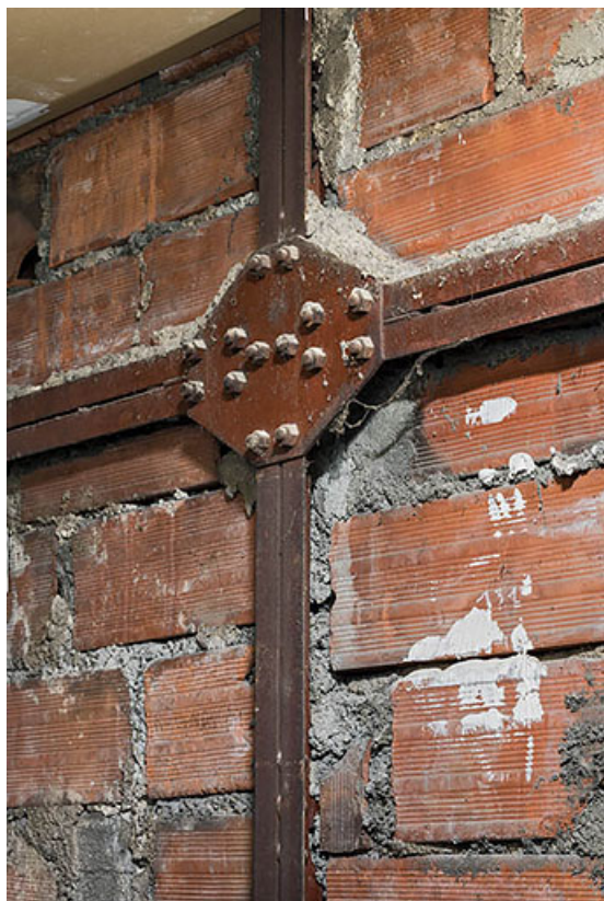
Détail du pan de fer d'un mur.
