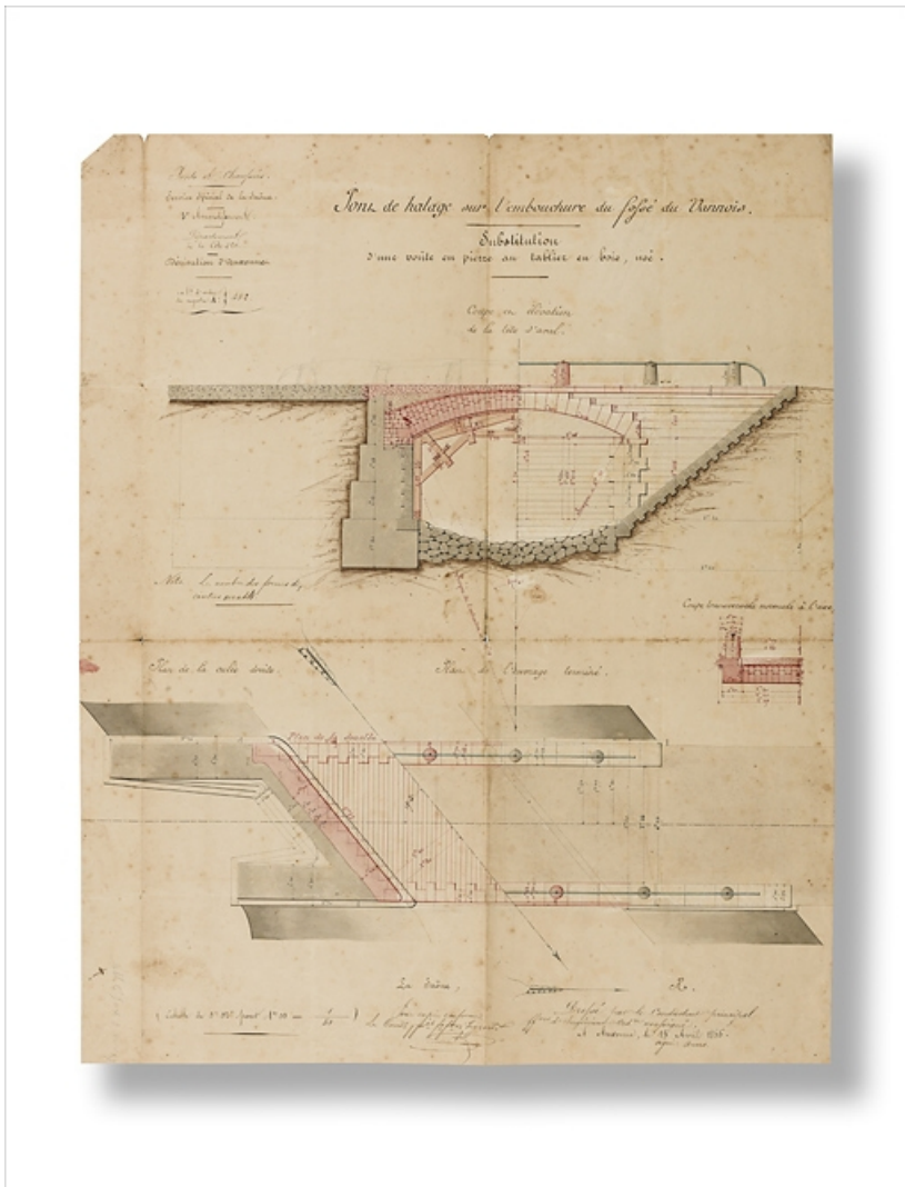
Pont de halage sur l'embouchure du fossé du Vannois. Substitution d'une voûte en pierre au tablier en bois, usé. 15 avril 1865. 21, Auxonne, lieudit : PK 229,5
