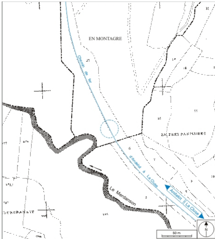
Plan-masse et de situation. Extrait du plan cadastral informatisé, 2006, section A, échelle 1:2000. 01, Arbent, lieudit : en Montagre
